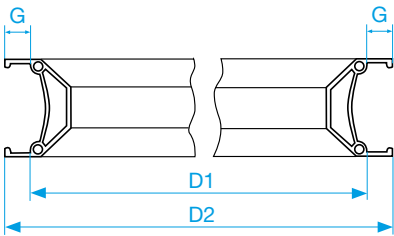
Tolleranza ETRTO per i cerchi a doppia camera
